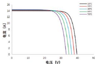
电流-电压曲线 SS8-54HD-420N
