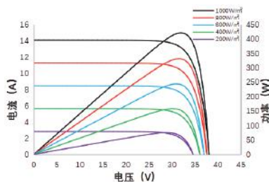
电流/功率-电压曲线 SS8-54HD-420N
