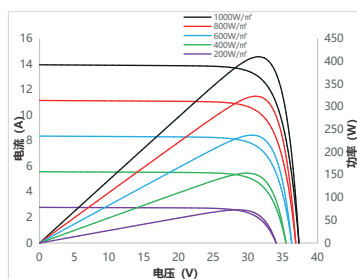
电流/功率-电压曲线 SS8-54HS -410M
