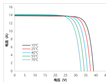
电流-电压曲线 SS8-54HS -410M
